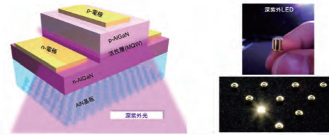
深紫外LEDデバイス構造
