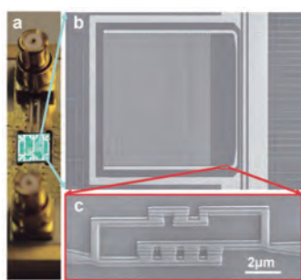
実際に用いた試料と回路素子 a. 試料ホルダーに装填された測定チップ b. 深強結合 qubit (赤枠箇所)-LC調和振動子回路、アルミニウム製 c. 超伝導 flux-qubit
