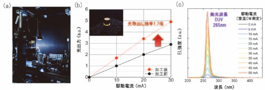
図4：(a) DUV-LEDを評価するために構築したシステム、(b) ナノ光取出し構造による DUV-LEDの出力性能の向上結果および (c) 各印加電流に対する発光スペクトル特性
