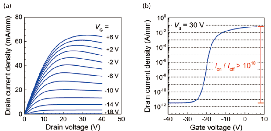
図4 Ga 2 O 3 MOSFETの (a) 出力特性、(b) トランスファ特性 この2つの図が示すように、Ga 2 O 3 MOSFETのデバイス特性は、パワートランジスタとして実用上要求される性能の多くを十分に満たすものだった。
