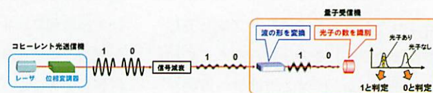
量子受信機の構成と原理
